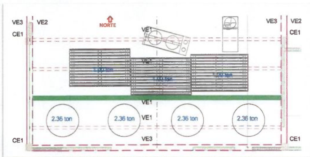
Vista en planta de techo con cargas de equipos y tinacos, imagen obtenida del Informe Preliminar Técnico Pericial de la edificación Jet Set Club.
