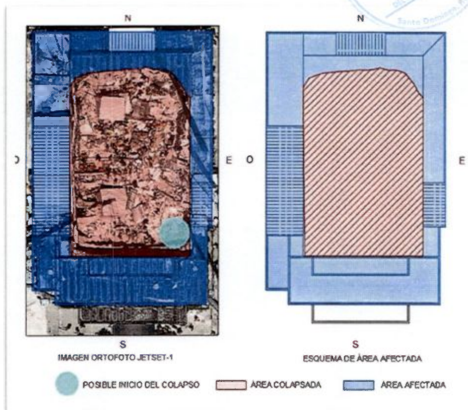
Esquema de área afectada de la edificación Jet Set Club, Imagen obtenida del Informe Preliminar Técnico Pericial de la edificación Jet Set Club.
