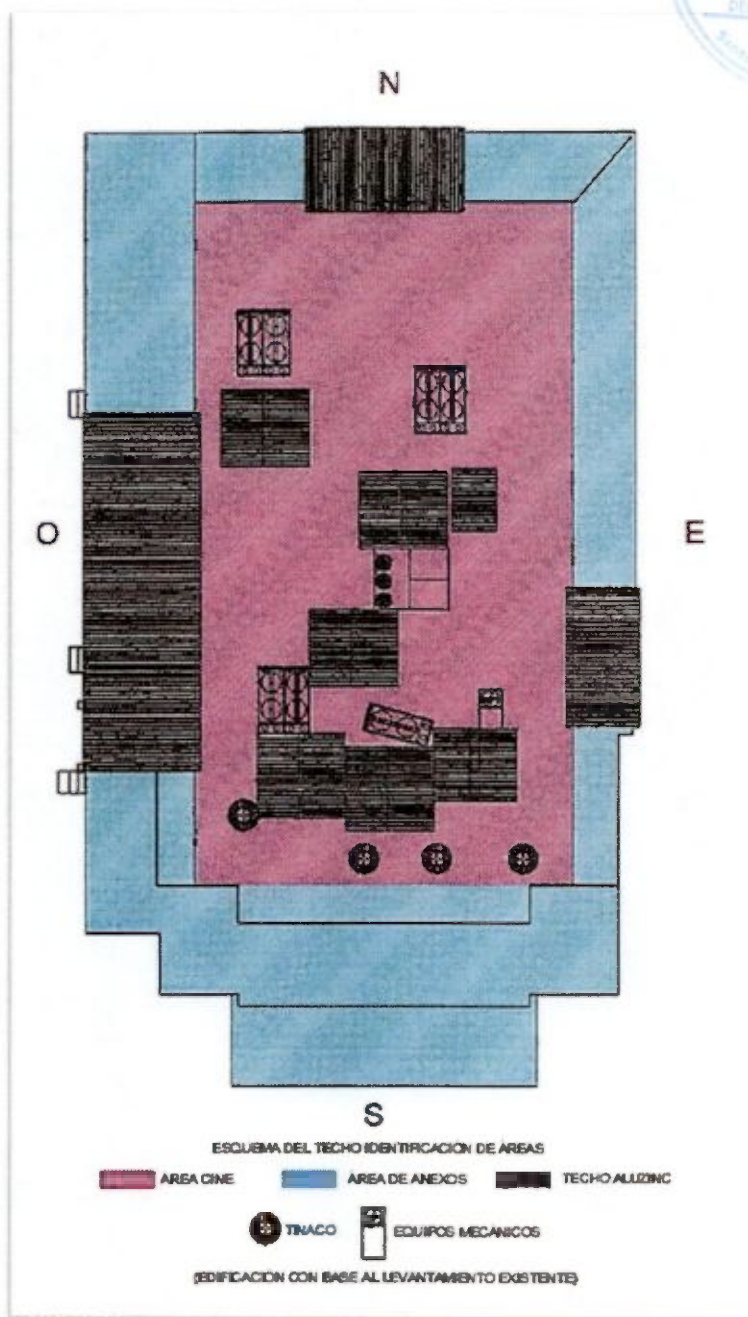
Esquema de elementos ubicados en el techo, imagen obtenida del Informe Preliminar Técnico Pericial de la edificación Jet Set Club.
